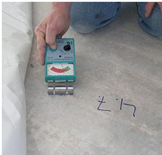
Weithin bekannt: das DNS-Feuchte-Meßgerät
